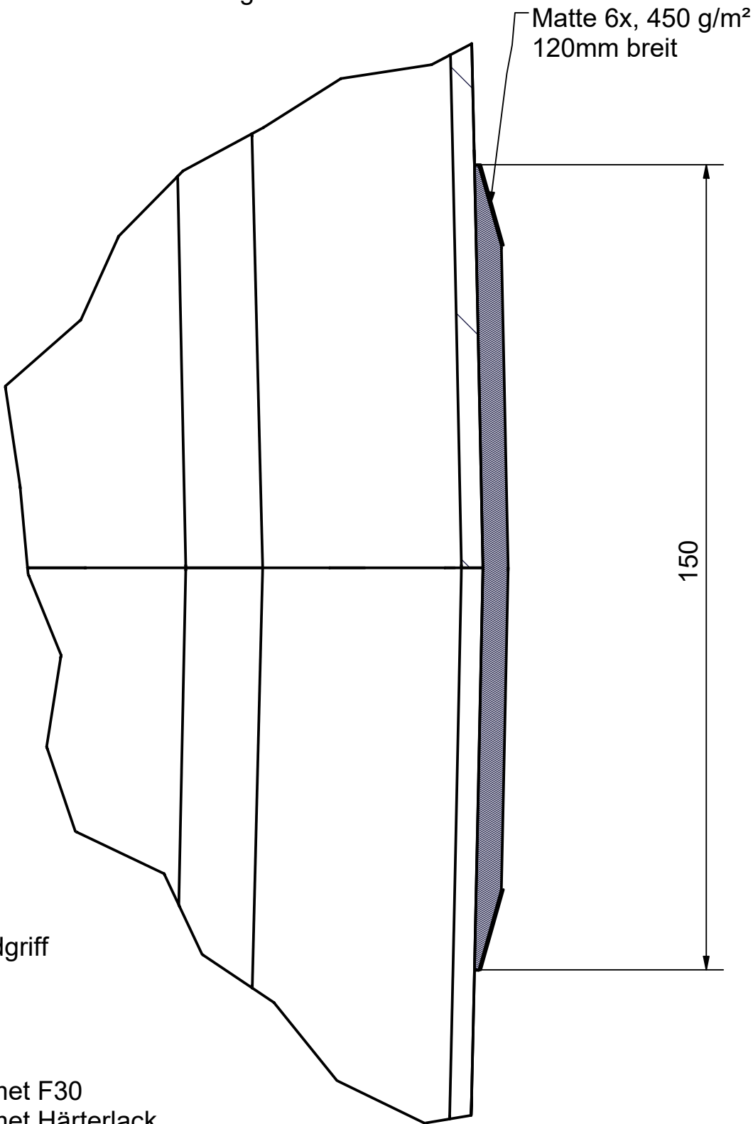
A - A ( 1 : 1 ) Verbindungsnaht
