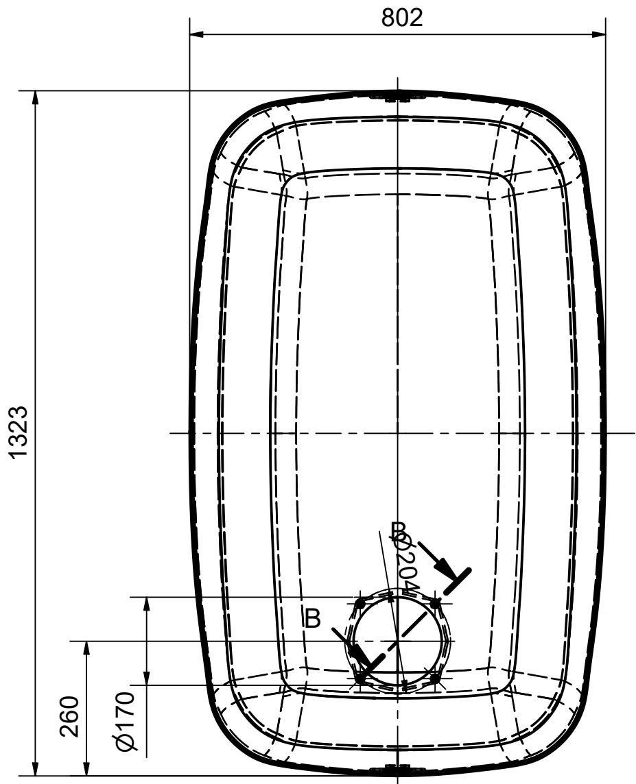
B - B ( 1 : 1 )
