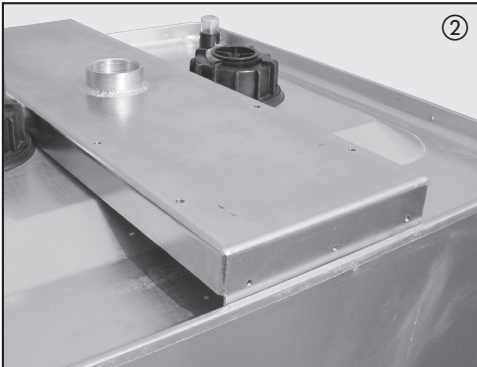
② Konsole mit 2" Muffe zentrisch über der Tanköffnung und innerhalb des Tankrandes platzieren.
