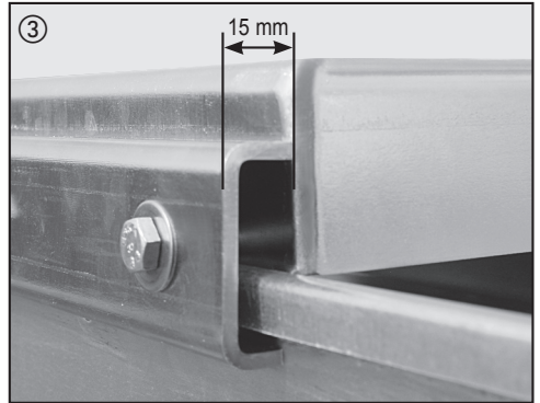
③ Klemmblech rechts/links mit Abkantung 15 mm an der Oberseite positionieren.
