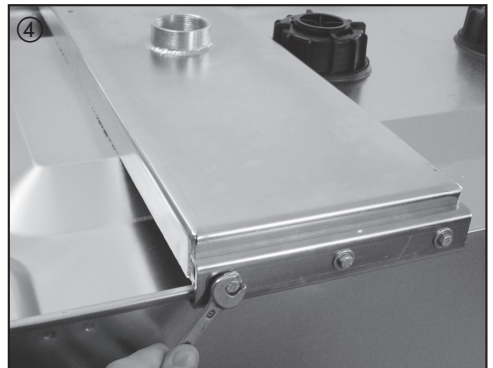
④ Klemmblech rechts/links mit jeweils 3 x 6kt-Schraube M6x25 am oberen Tankrand festschrauben.
