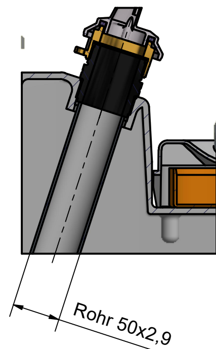
A-A (1 : 4)
