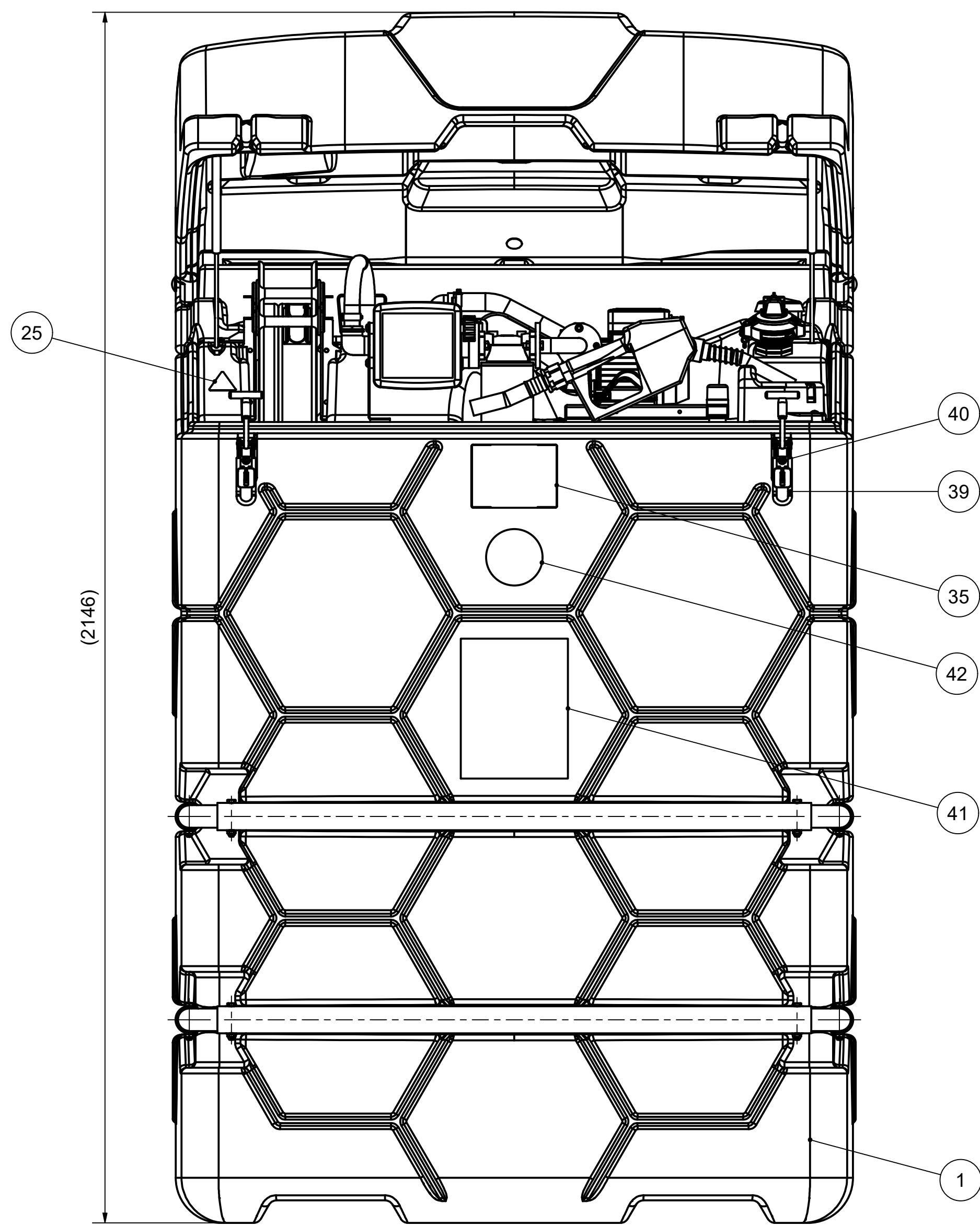
Draufsicht ohne Klappdeckel
