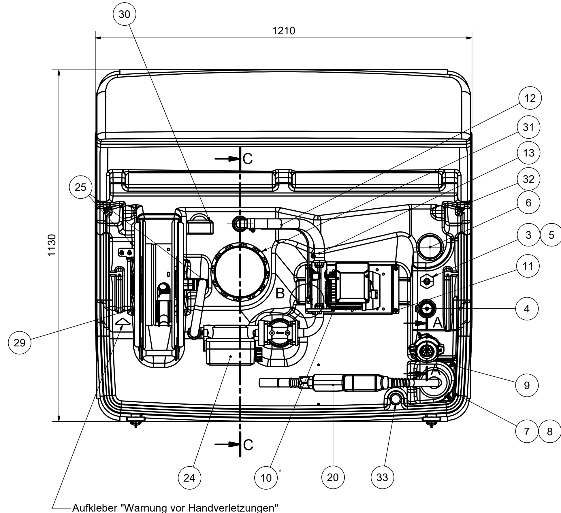
Draufsicht ohne Klappdeckel
