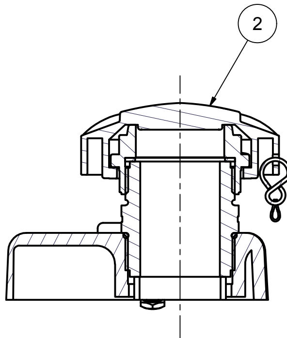
A-A ( 1 : 2 )
