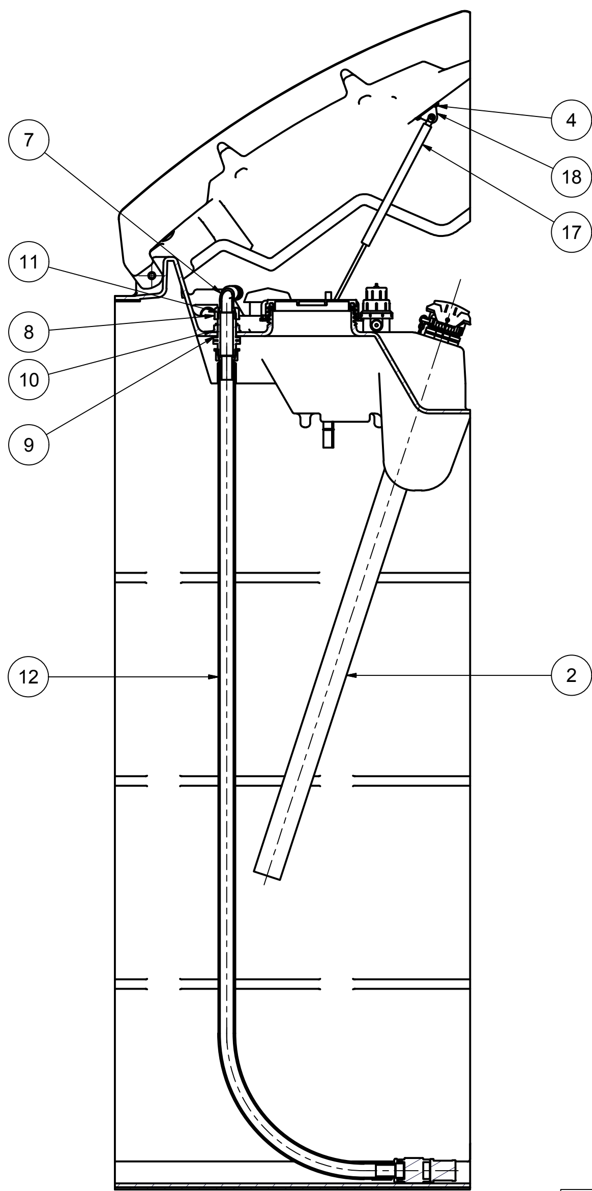
C-C ( 1 : 7 )
