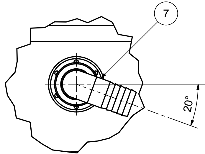
B ( 1 : 2 )
