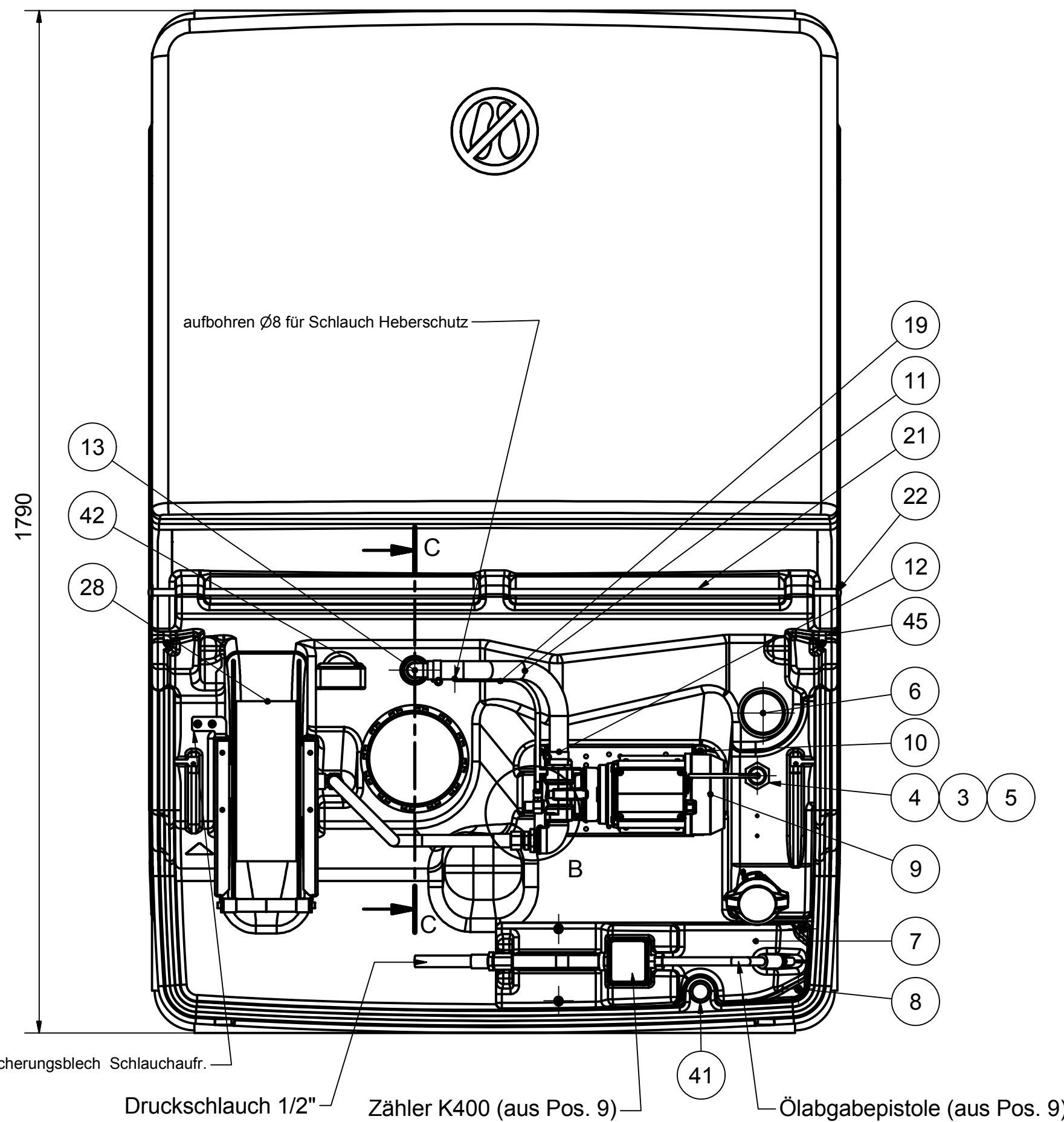
Draufsicht ohne Klappdeckel
