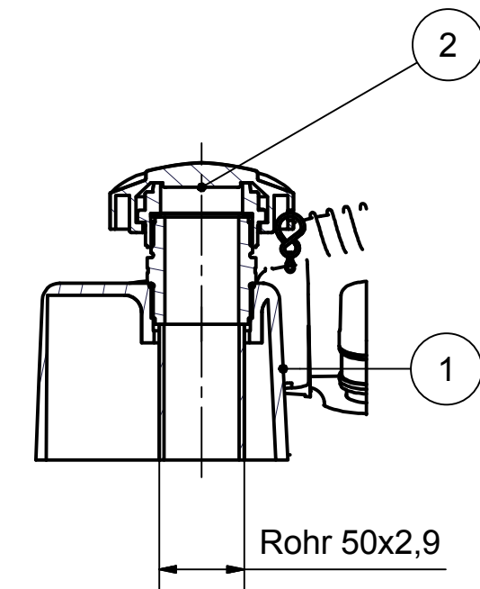
A-A ( 1 : 4 )
