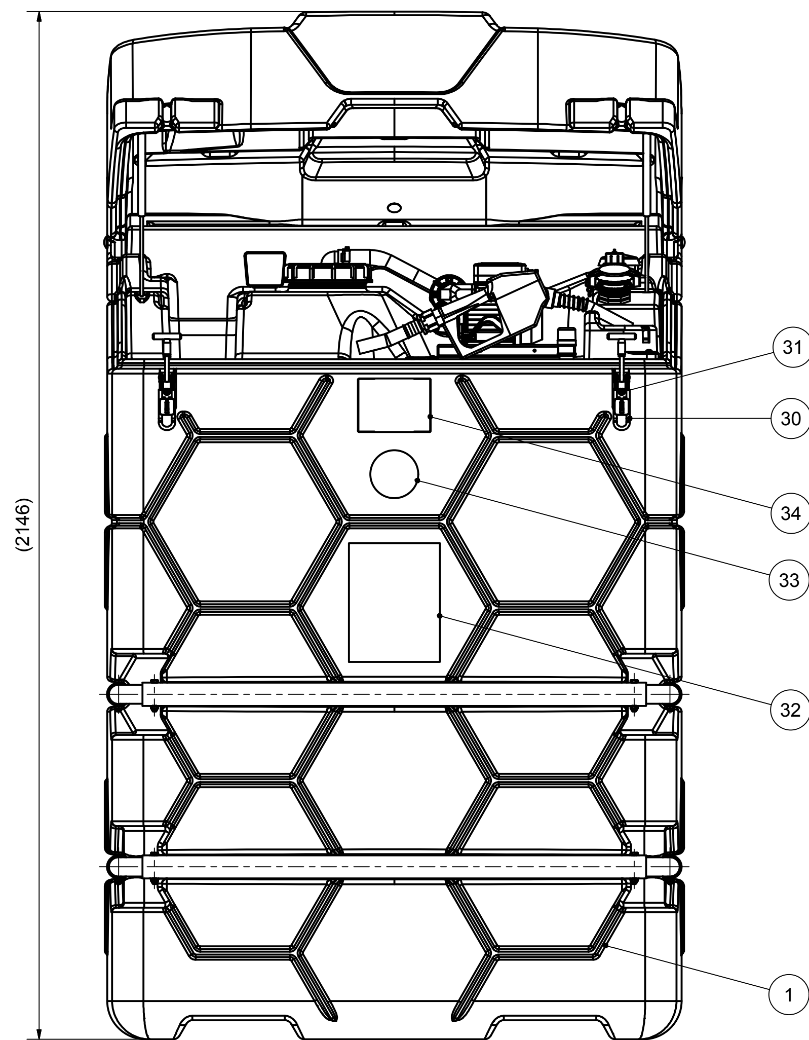
Draufsicht ohne Klappdeckel
