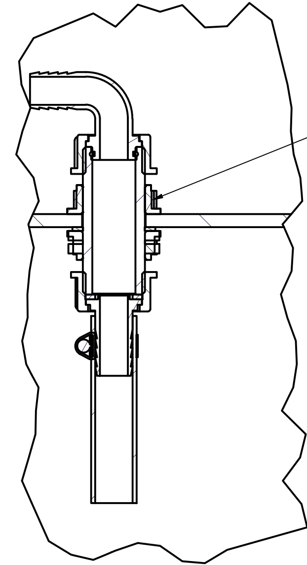
B ( 1 : 2 )
