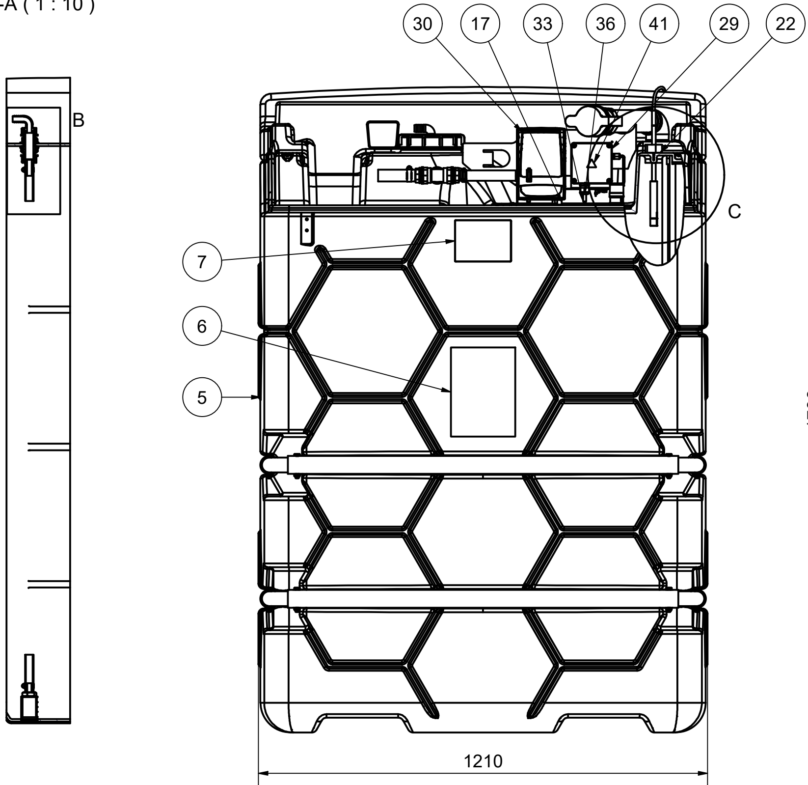
A-A ( 1 : 10 )
