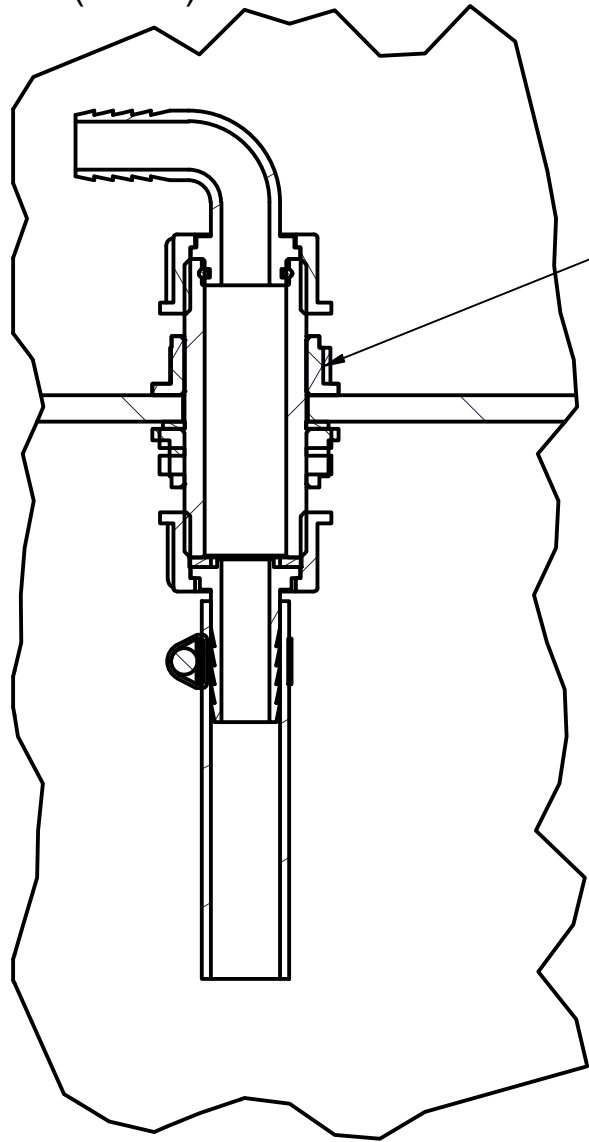
B ( 1 : 2 )
