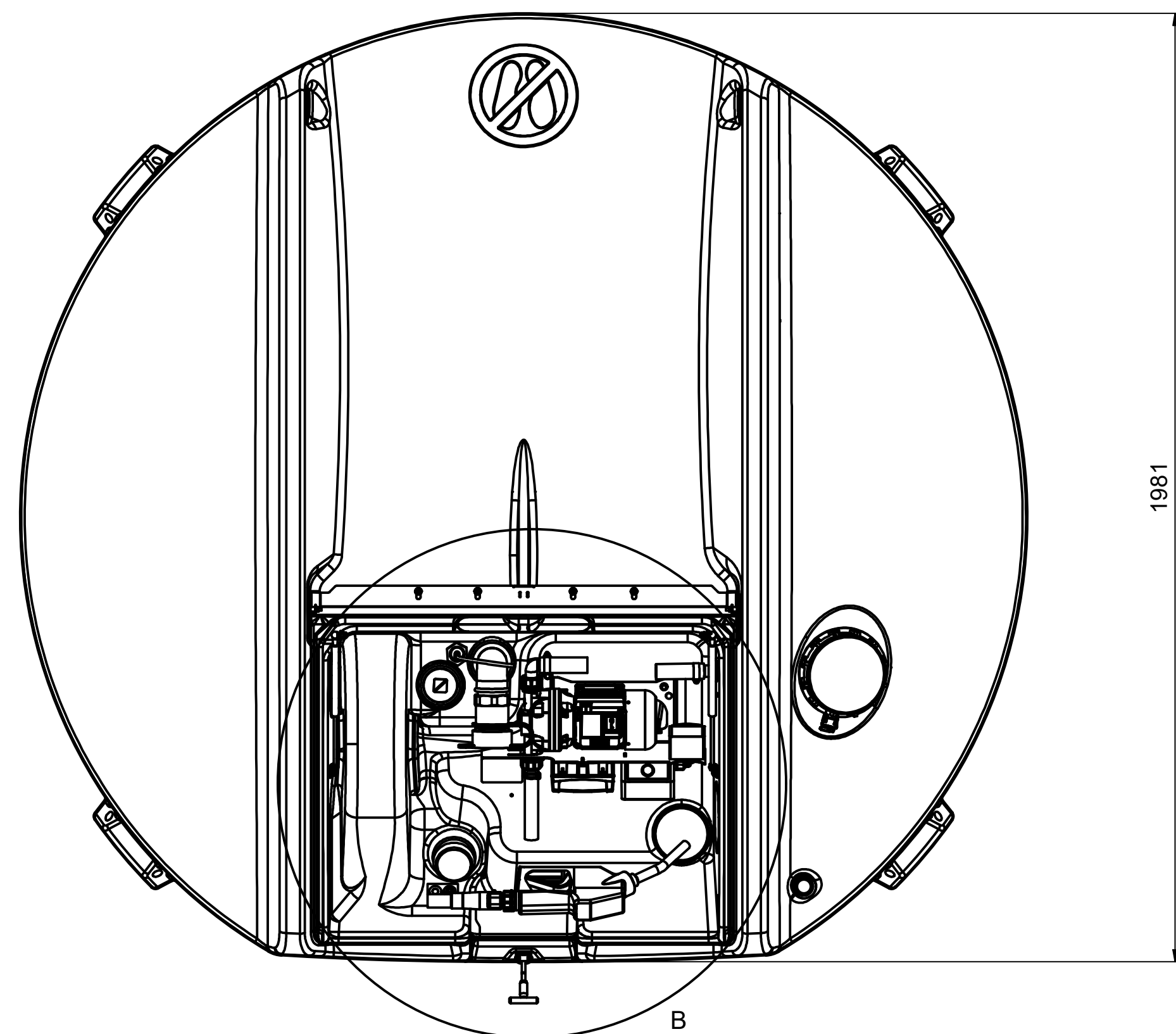
Darstellung ohne Klappdeckel ( 1 : 10 )
