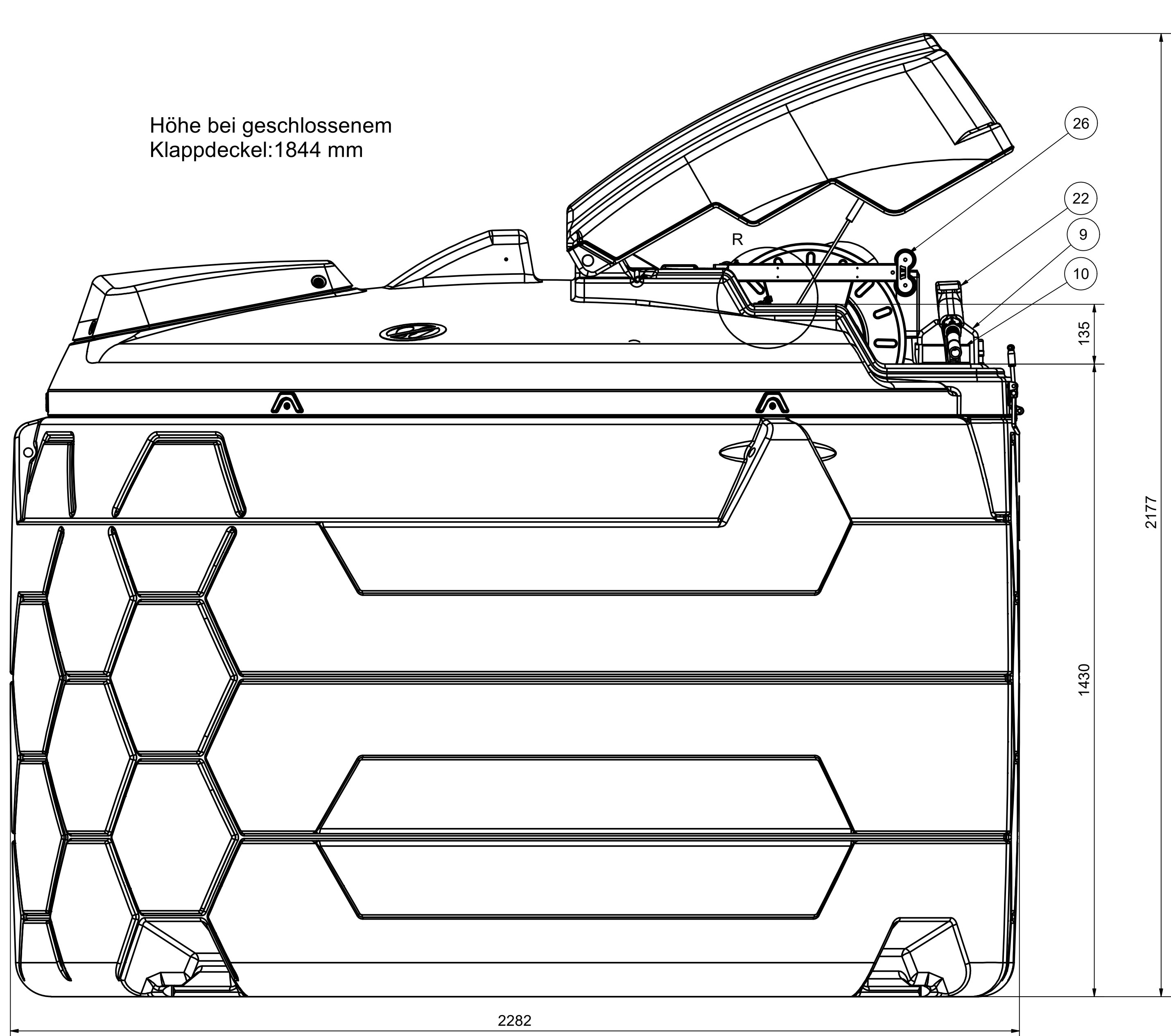
A-A ( 1 : 6 )
