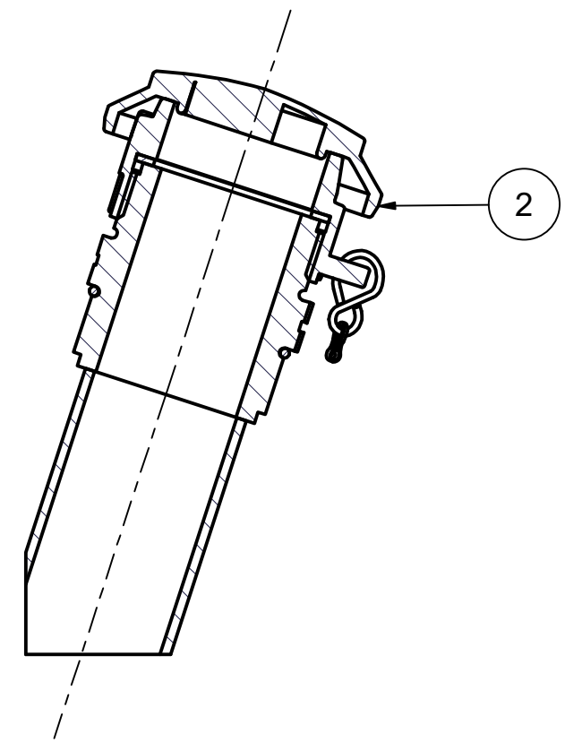
B-B ( 1 : 2 )
