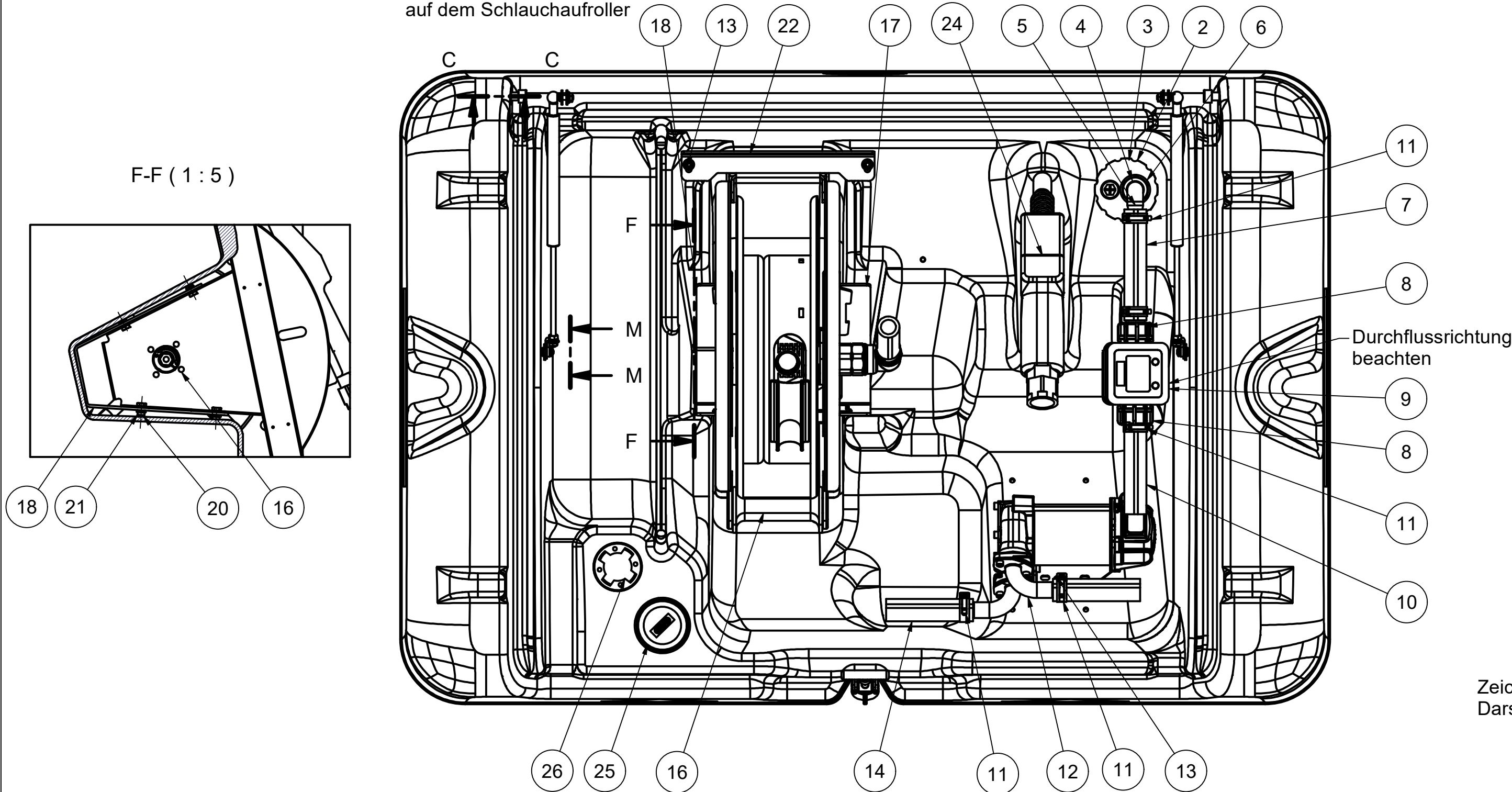
Draufsicht ohne SMC-Deckel dargestellt ohne Schlauch auf dem Schlauchaufroller
