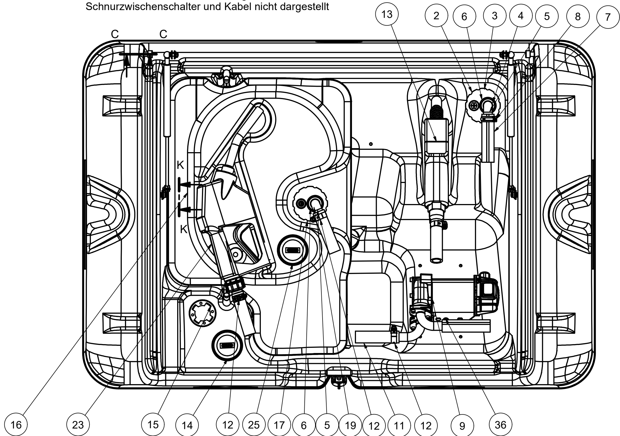
Draufsicht ohne SMC-Deckel dargestellt Schnurzwischenschalter und Kabel nicht dargestellt
