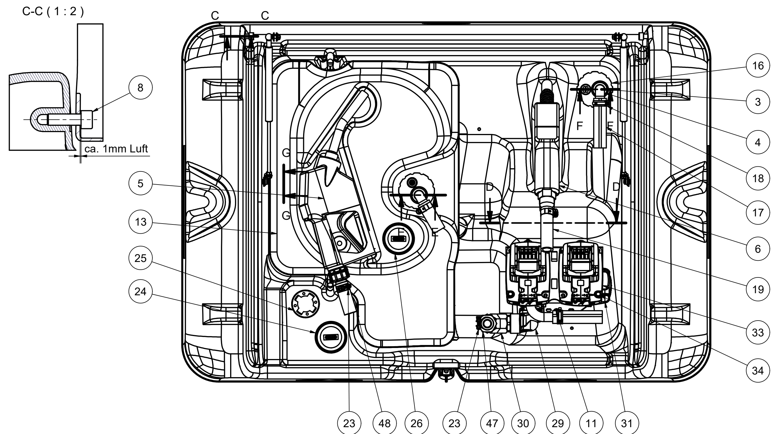
Draufsicht ohne SMC-Deckel dargestellt
