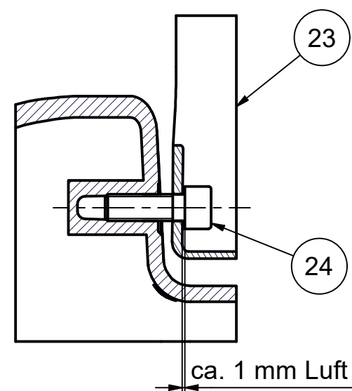
C-C (1:2)
