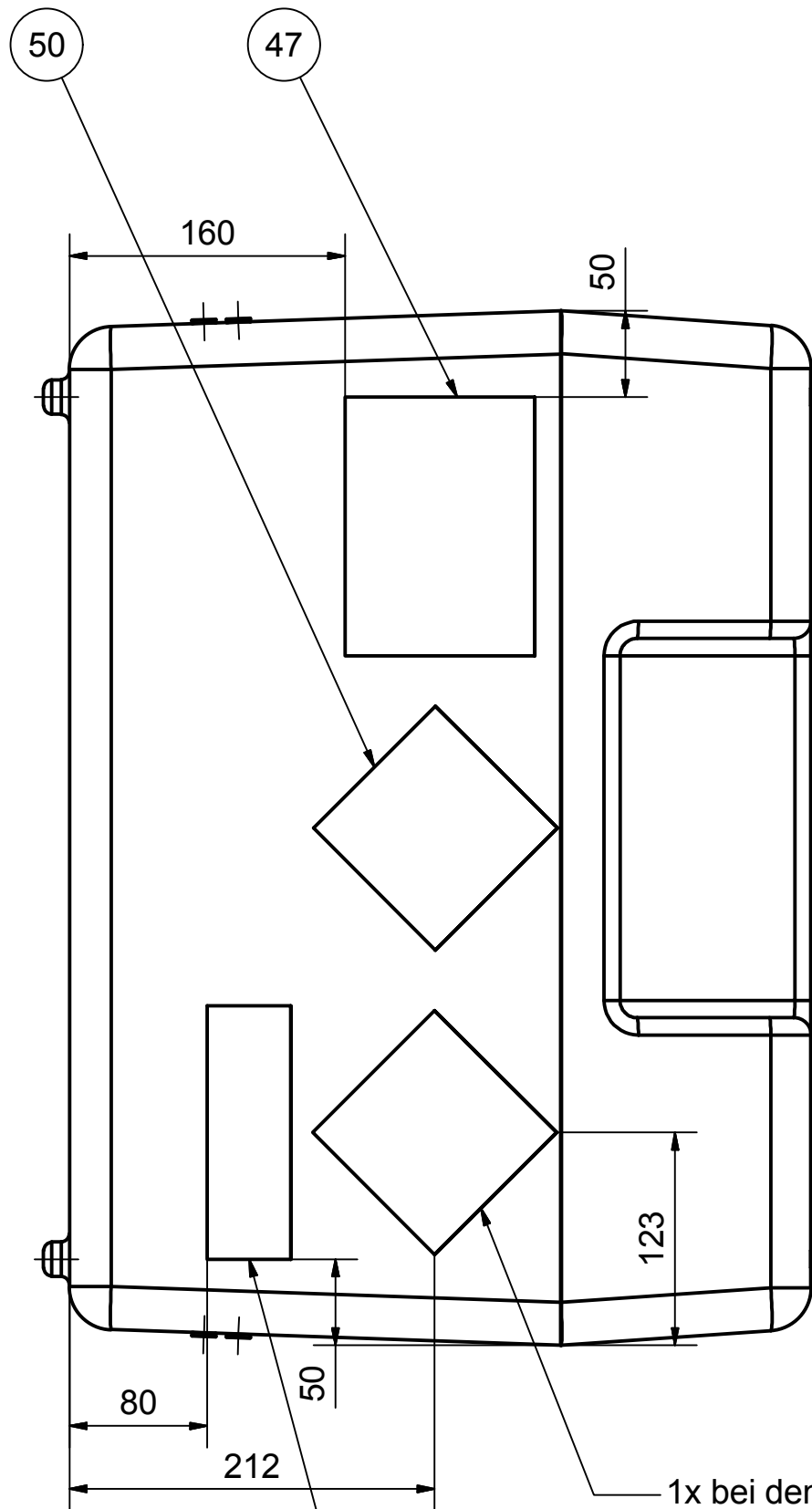
Knickschutzfeder gek. dargestellt
