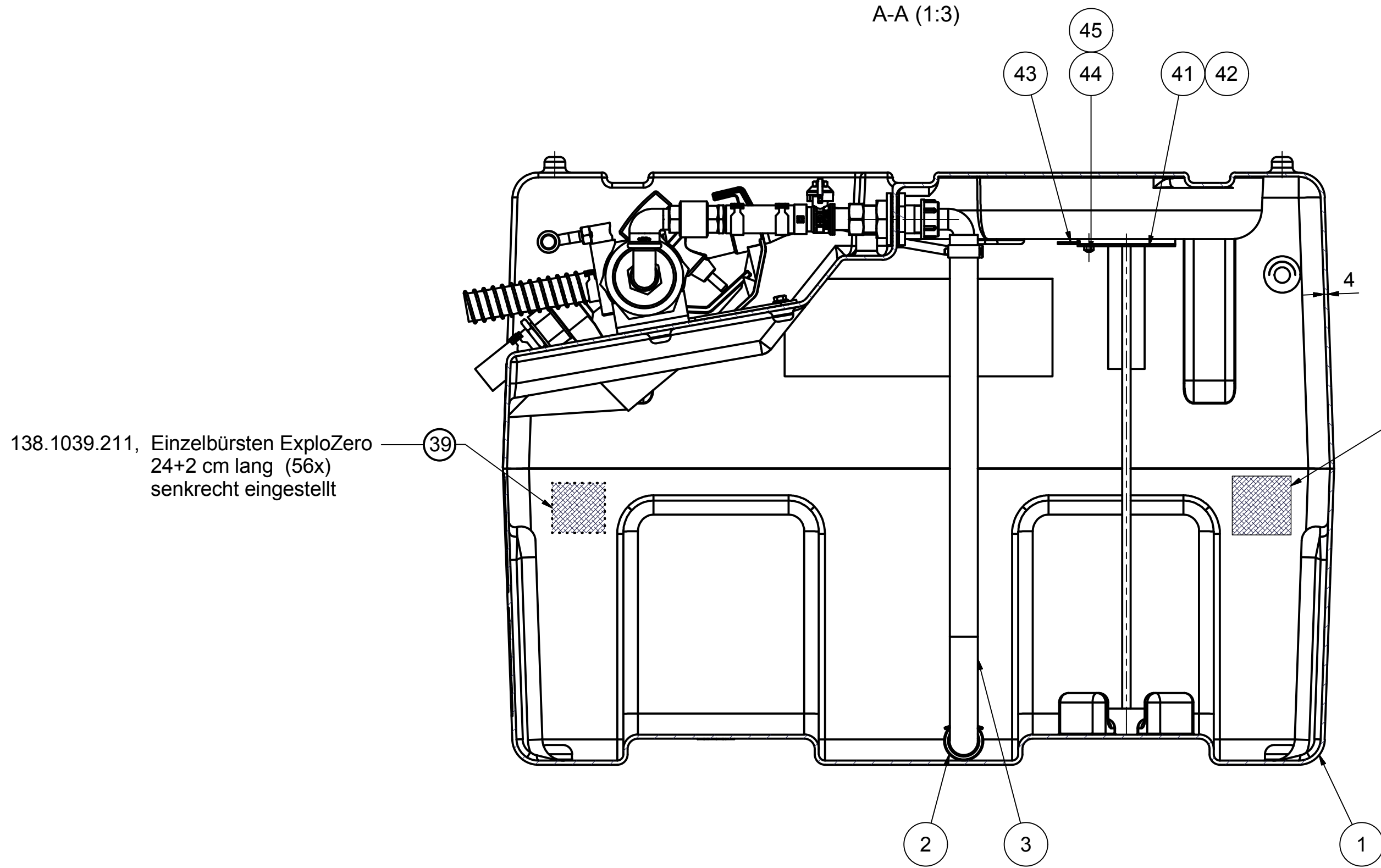
A-A (1:3)
