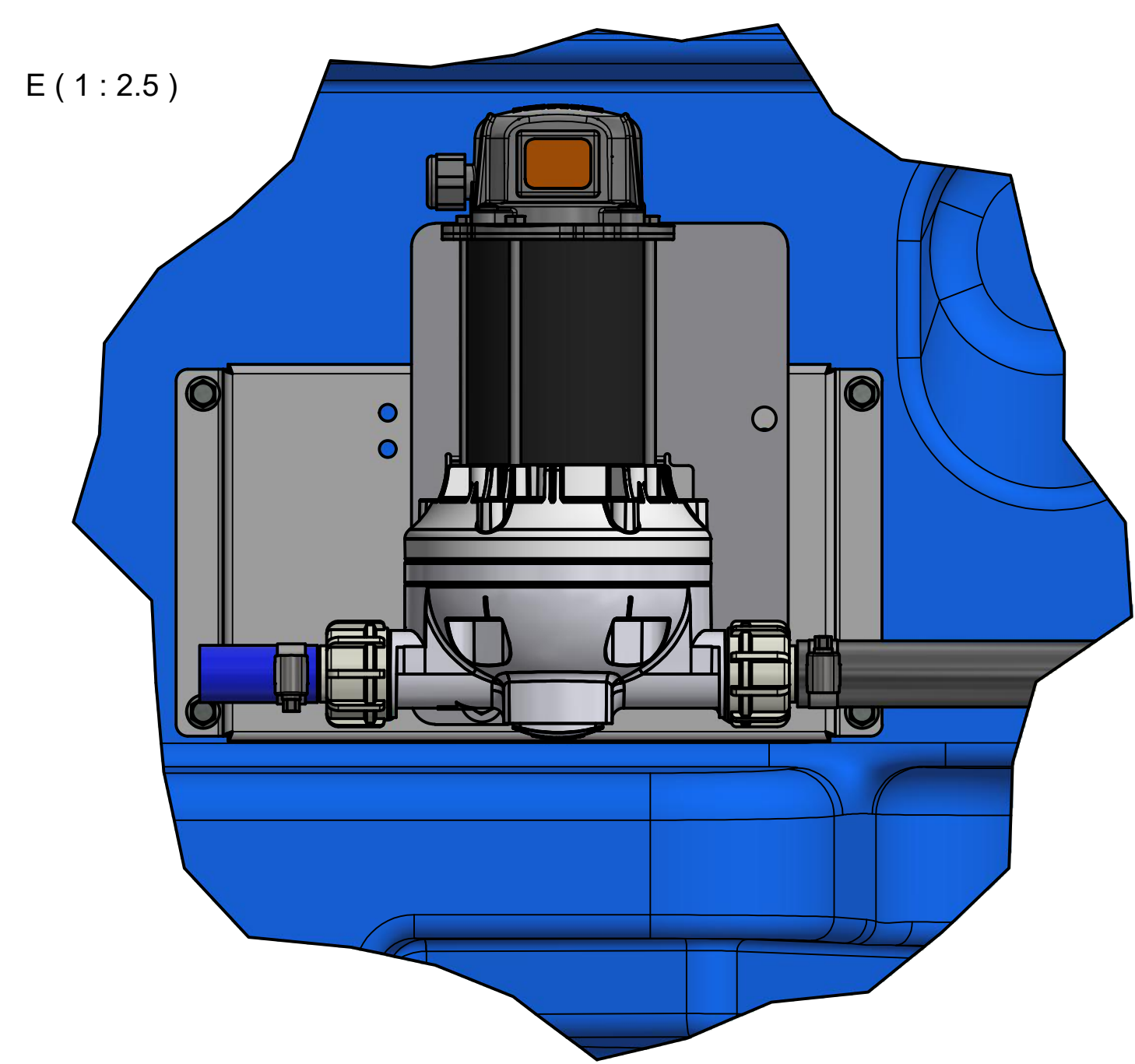
Darstellung mit 936.2931.035 Cematic Blue 12 V mit Adapterblech Saugschlauchlänge 0,18 m
