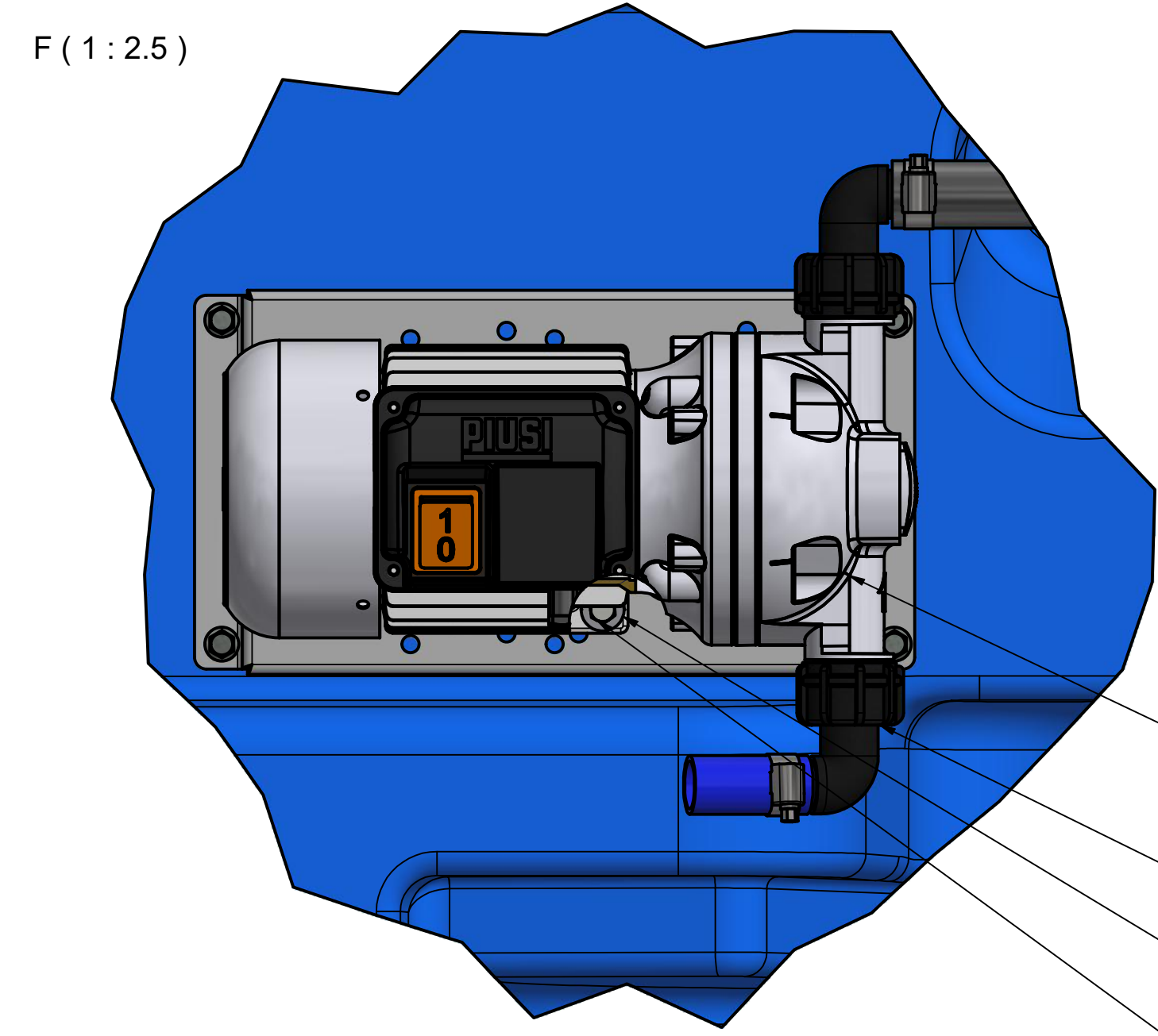
Darstellung mit 936.2910.035 Cematic Blue 230 V mit Adapterblech Saugschlauchlänge 0,4 m
