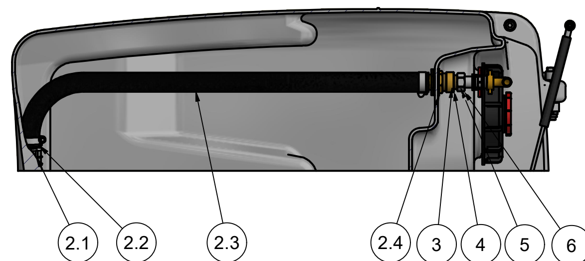
A-A (1:7)
