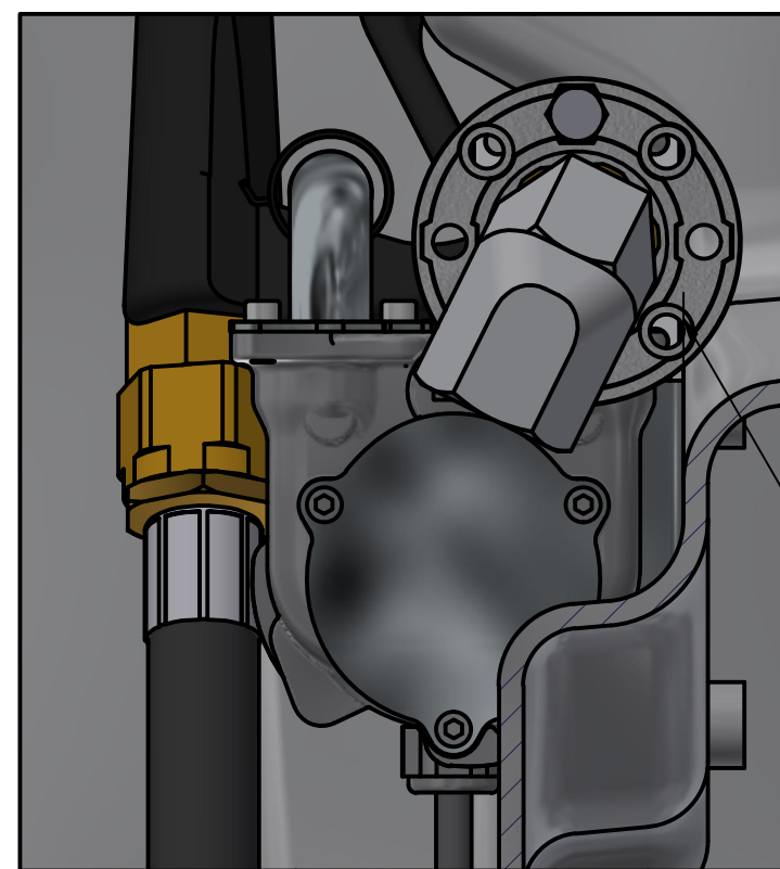
G-G (1:2)
