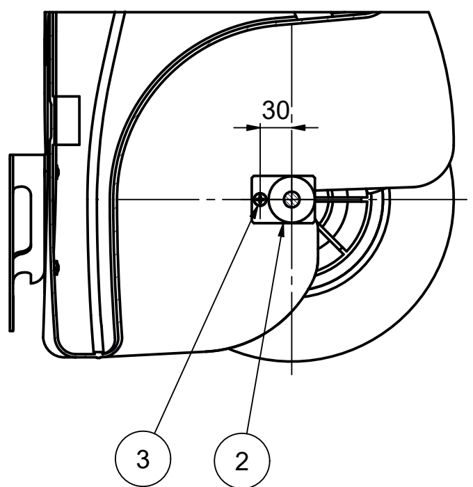
E-E ( 1 : 5 )
