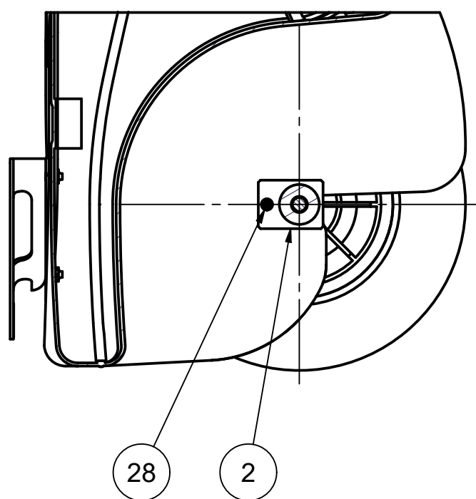
D ( 1 : 1 )
