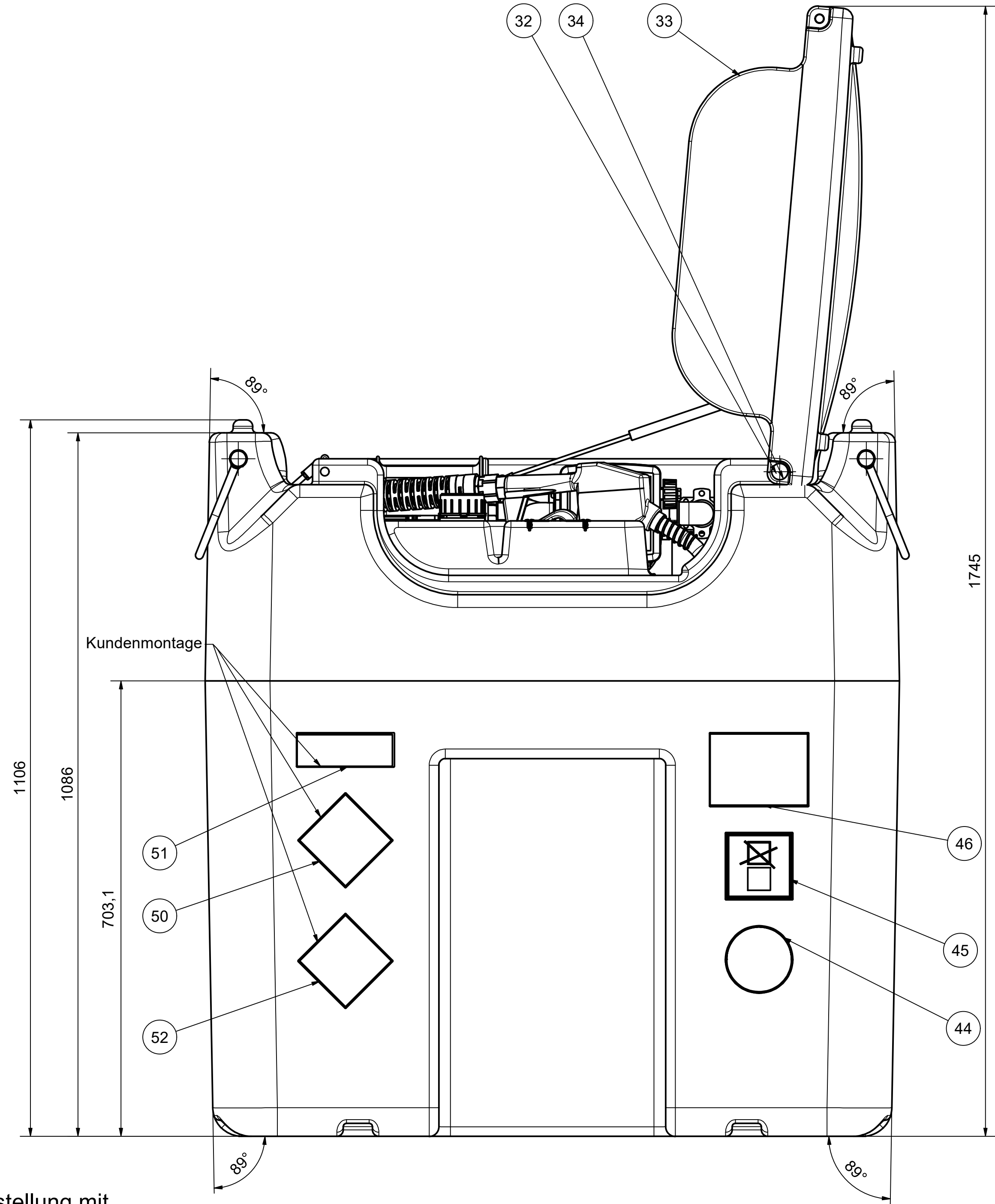
Darstellung mit 138.1719.208 E-Pumpe Cematic 72 m. Adapterblech
