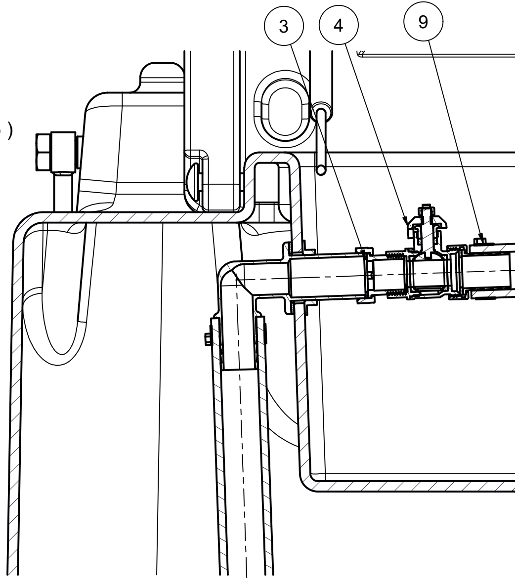
A-A (1:2.5)
