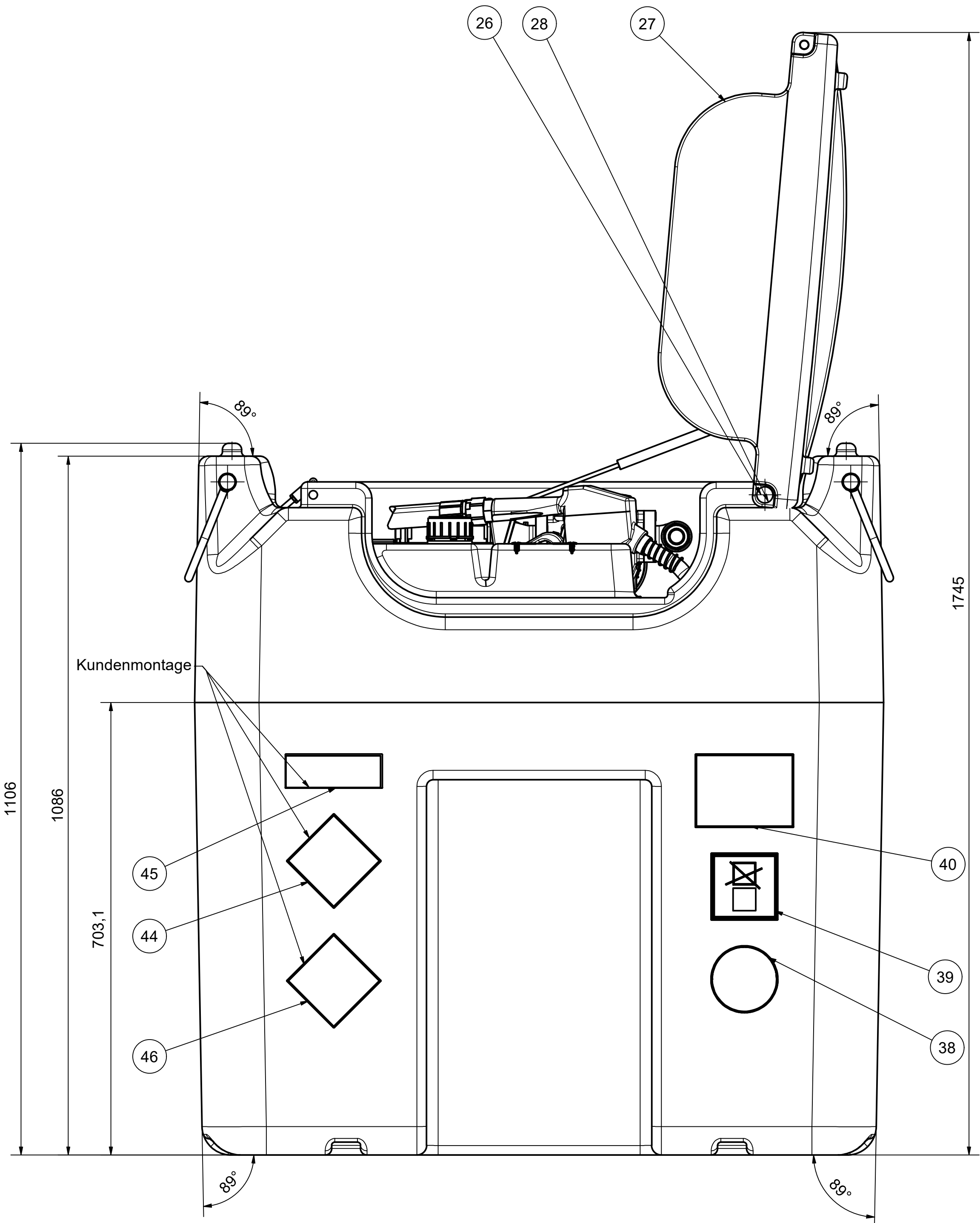
138.1617.003 DT Mobil Easy 980 Darstellung mit 138.1719.208 E-Pumpe Cematic 72 m. G (1:2.5) Adapterblech
