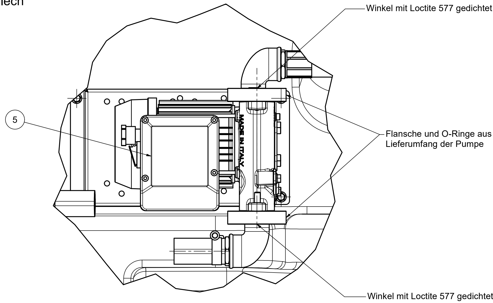
138.1617.003 DT Mobil Easy 980 Darstellung mit 138.1719.208 E-Pumpe Cematic 72 m. G (1:2.5) Adapterblech
