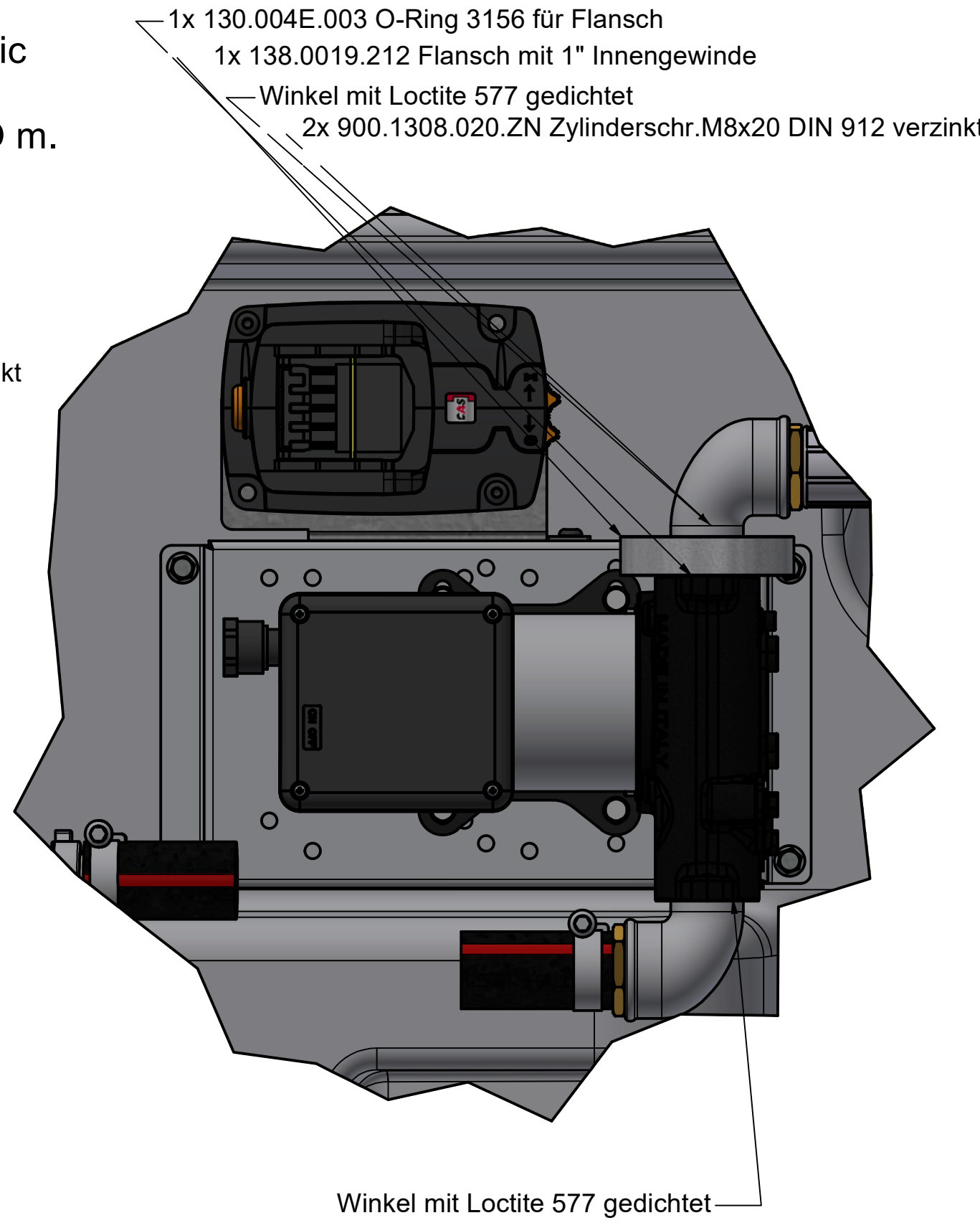
138.1616.006 DT Mobil Easy 980 Basic Cematic 56/18 Darstellung mit 138.1719.295 E-Pumpe Cematic 56/18 m. Adapterblech
