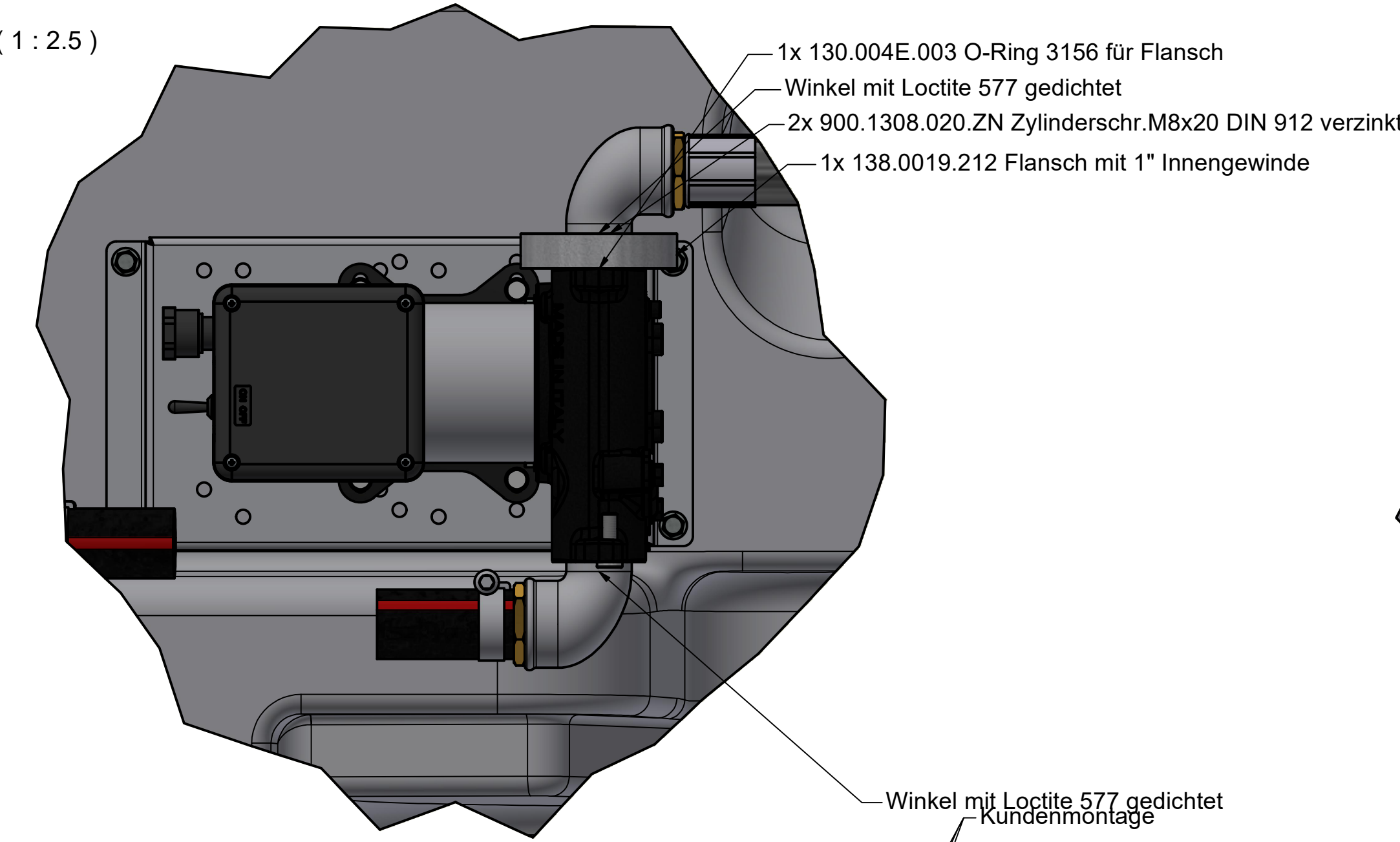
138.1616.003 DT Mobil Easy 980 Basic Darstellung mit 138.1719.211 E-Pumpe Cematic DUO m. Adapterblech
