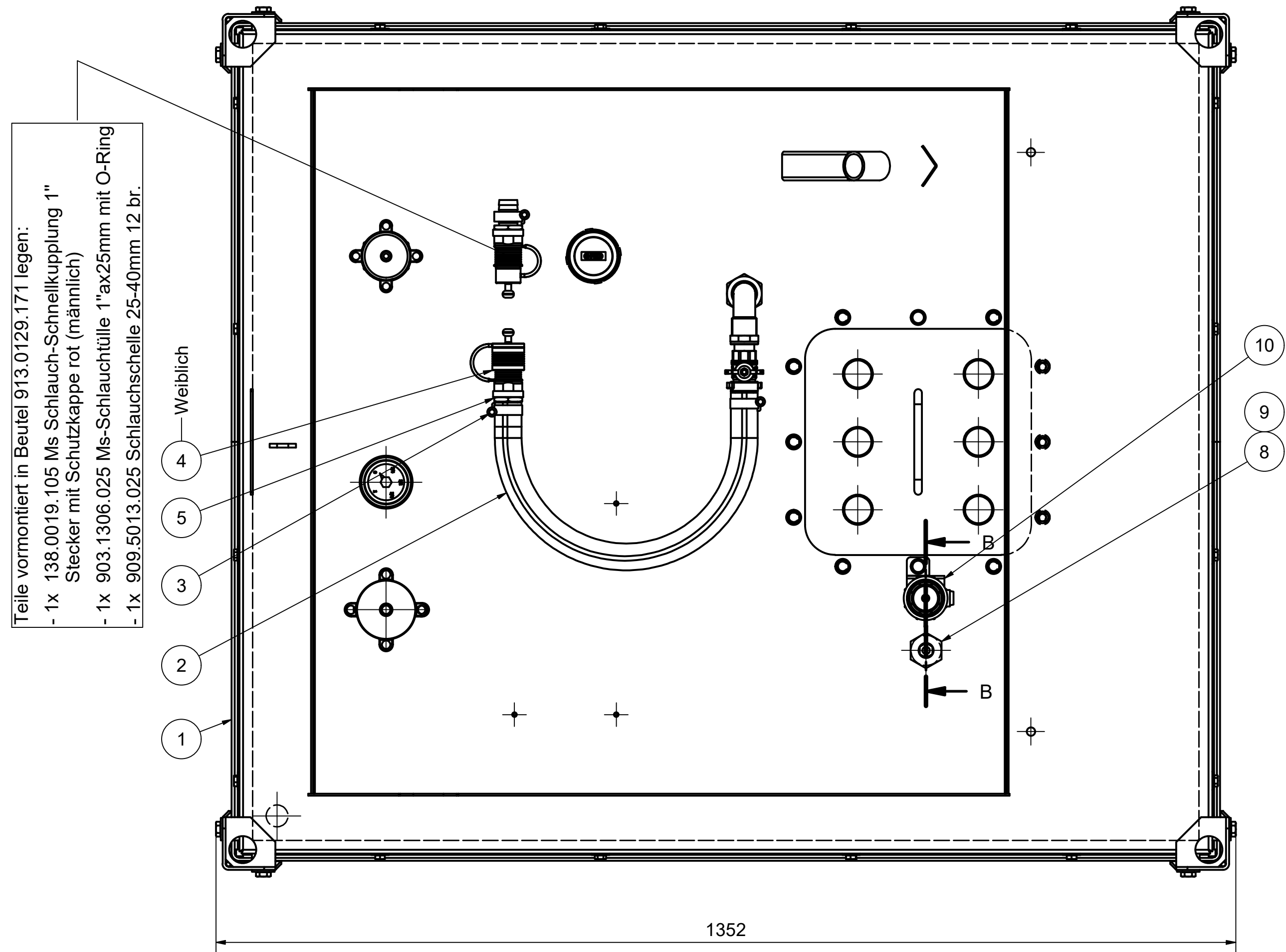
DRAUFSICHT ( 1 : 5 ) ohne Klappdeckel und Schließmechanismus dargestellt
