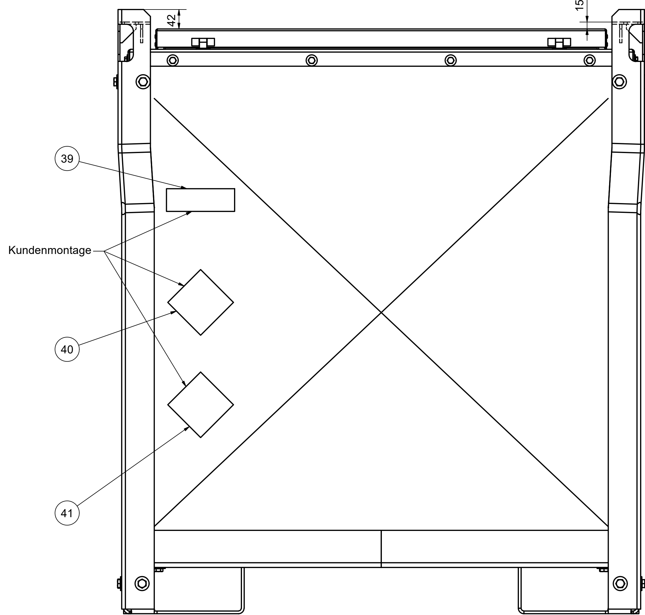
RÜCKSEITE (1 : 5) mit geschlossenem Klappdeckel dargestellt
