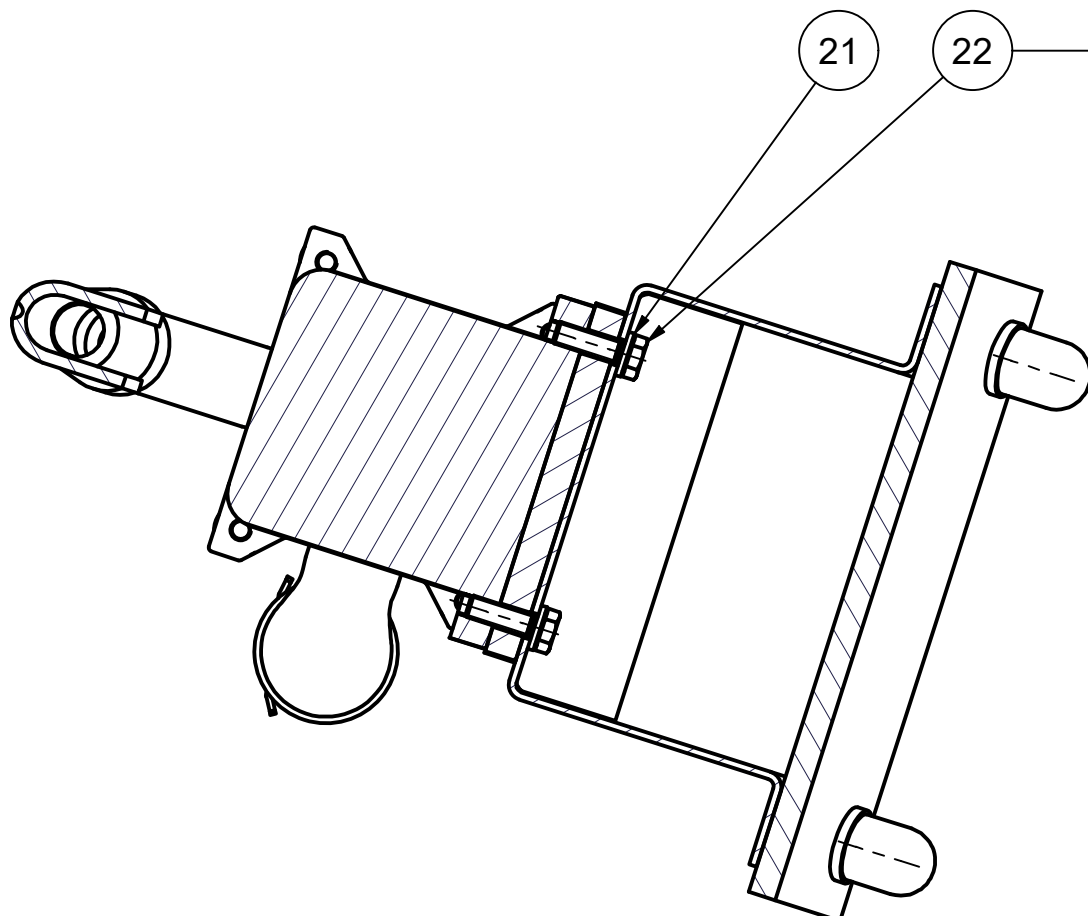
F-F (1 : 2)
