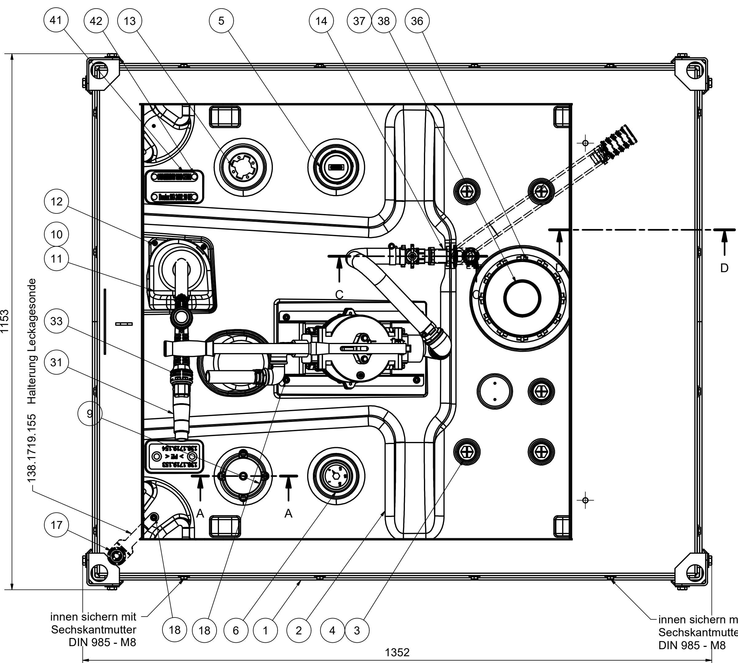
DRAUFSICHT (1 : 5) ohne Klappdeckel und Schließmechanismus dargestellt
