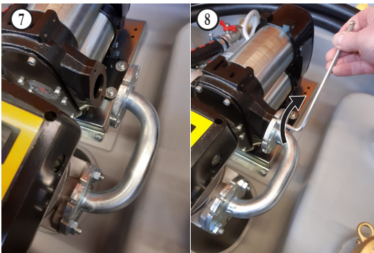
Anbau des kompletten Zählwerks.
