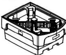
Typ 4 (Einfachstation mit Abfüllvorsatz und Stützkreuz, 1000 l)
