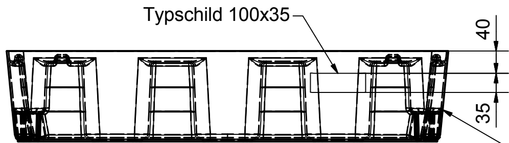
211.5509.003, PE-Auffangwanne 60 HD 80 x 60 x 16,5 cm, Spritzgussteil
