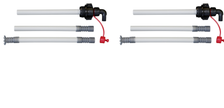
10872 - Saugrohr mit Kupplung AF2, S70x6 mit Schlauchtülle DN 19, 90grd
