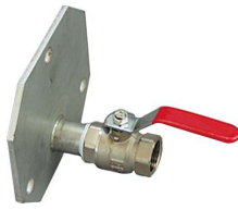
1319 - MS-Auslaufhahn 1" m.Flansch 100mm
