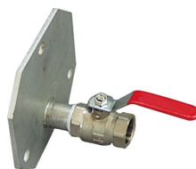
1326 - Kugelhahn Ms-vern. 3" mit Edelstahlflansch ab 1600I
