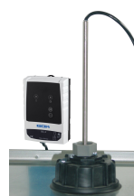
11452 - Ueberfuellsicherung BC-2 kpl., IP 54 mit Sonde 500 mm und Kabel 3 m
